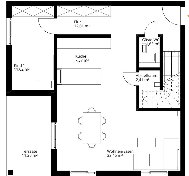
Erdgeschoss
