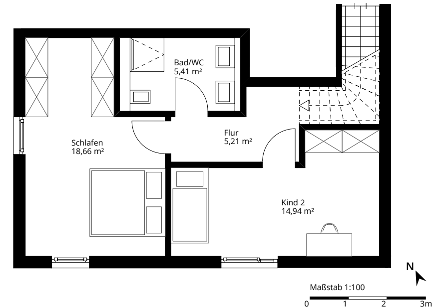
Obergeschoss
