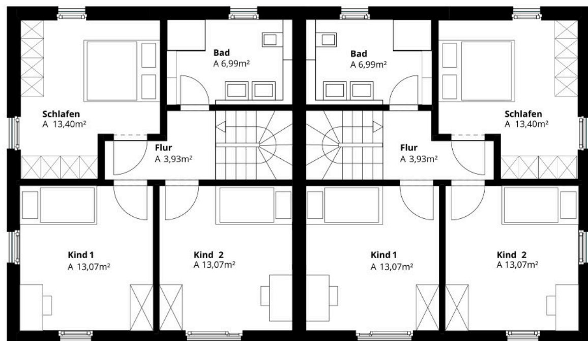
Obergeschoss
