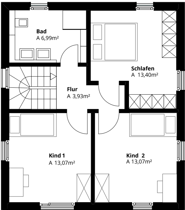
Obergeschoss
