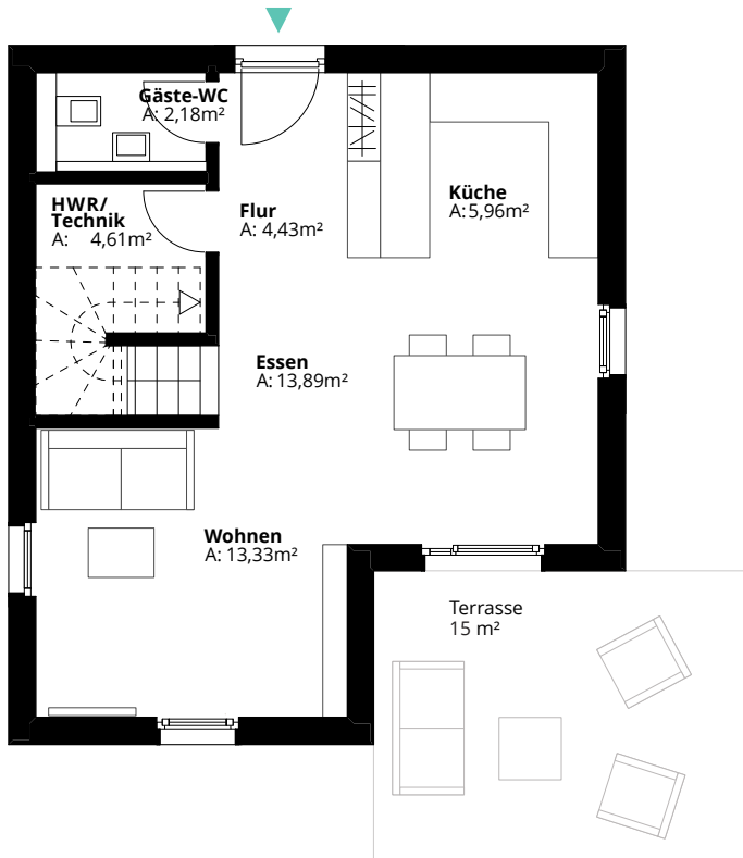
Erdgeschoss
