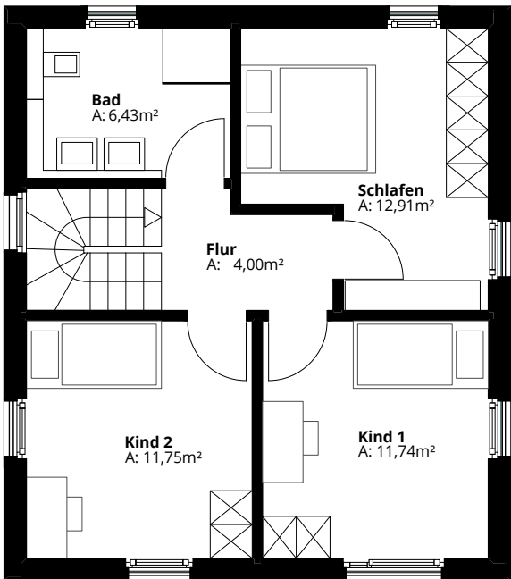
Obergeschoss
