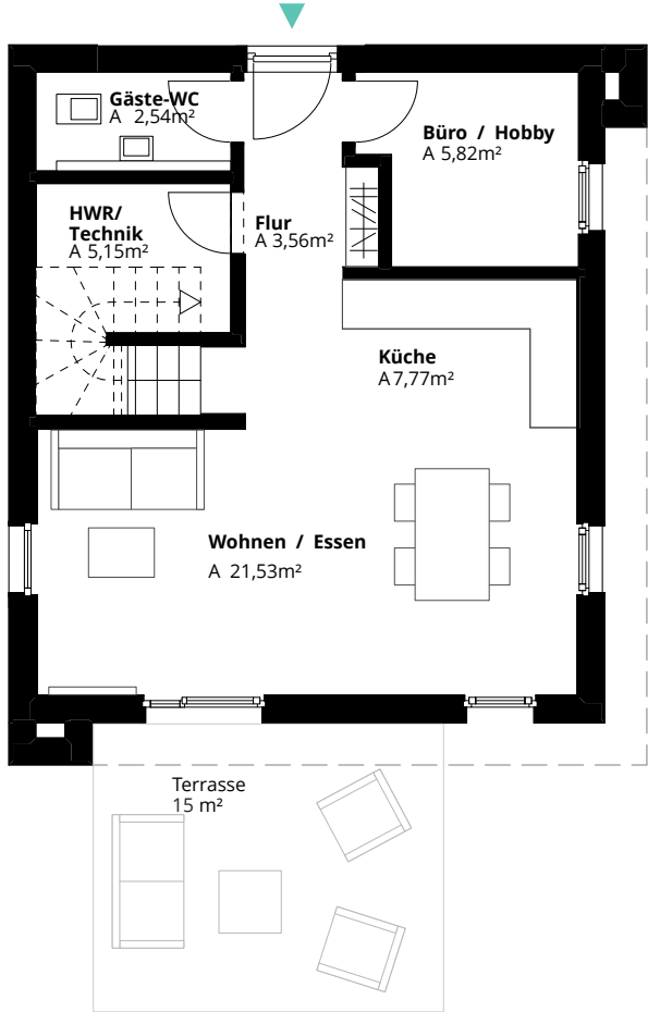
Erdgeschoss
