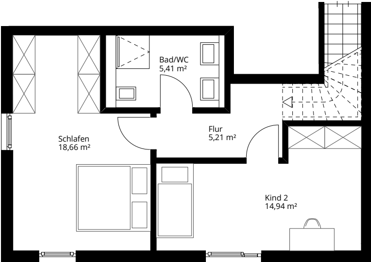
Obergeschoss
